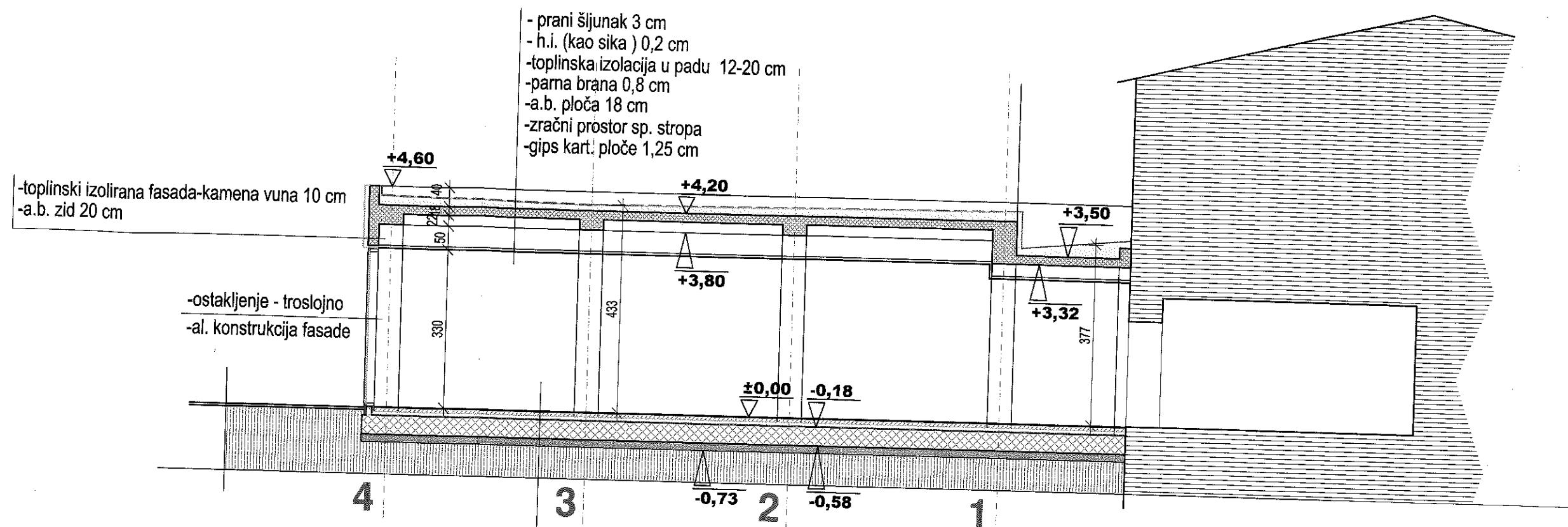
PRESJEK 1-1
